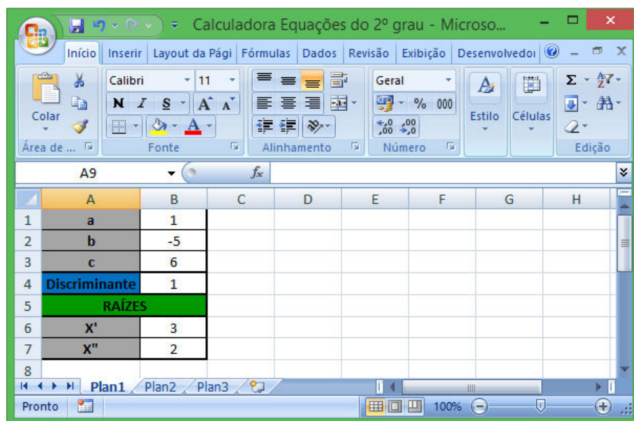
Figura 3 – Cálculo das raízes da equação x^2 - 5x + 6 = 0 usando planilhas eletrônicas
