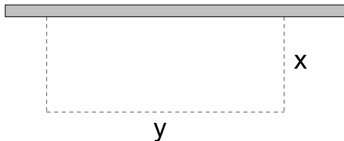
Figura 4 – Representação do cercado a ser construído
