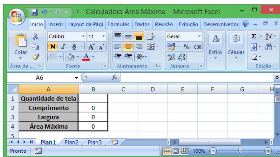
Figura 5 – Calculadora das dimensões do cercado de área máxima
