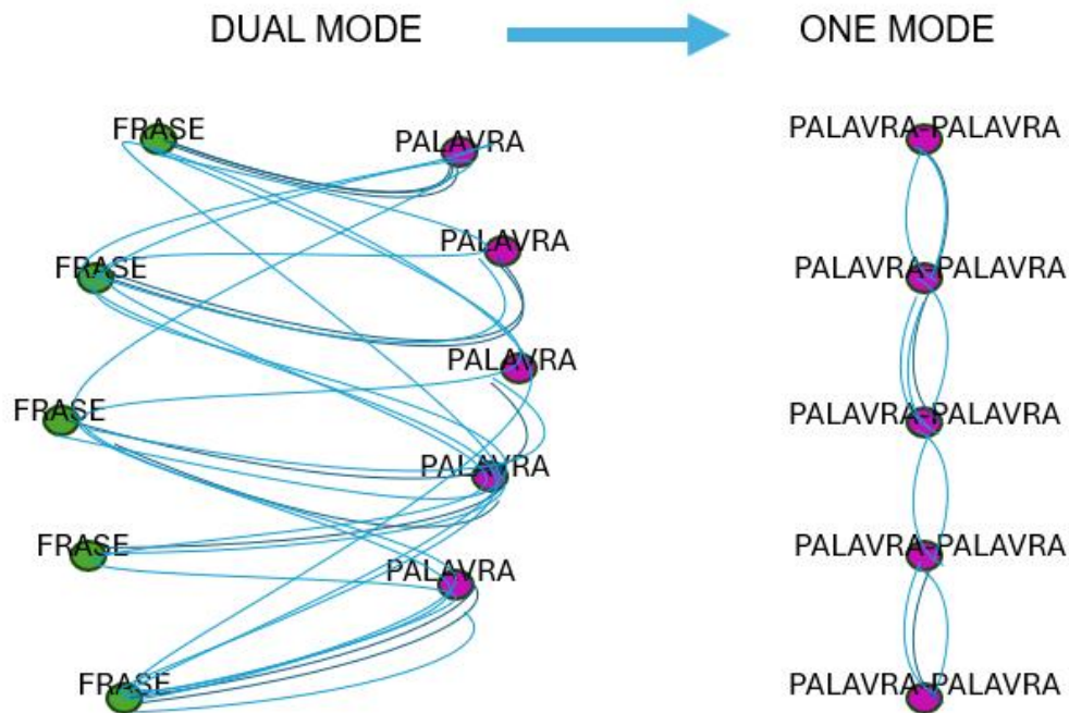
Figura 11 – Exemplo de projeção dual mode/one mode
