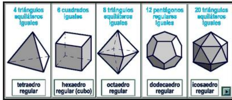
Figura 3.9: Poliedros regulares
