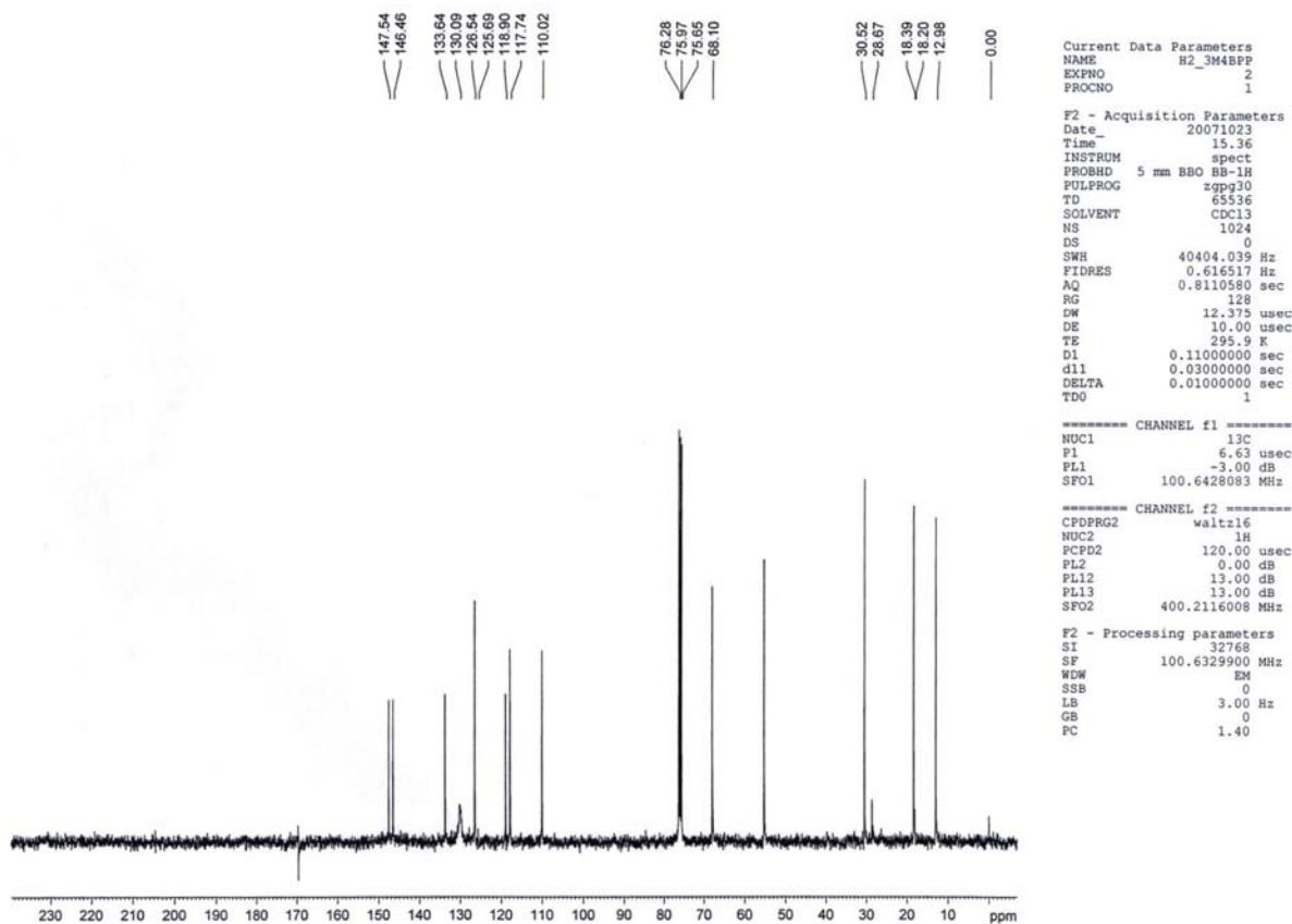
Espectro de RMN 13 C a 100 MHz de 27
