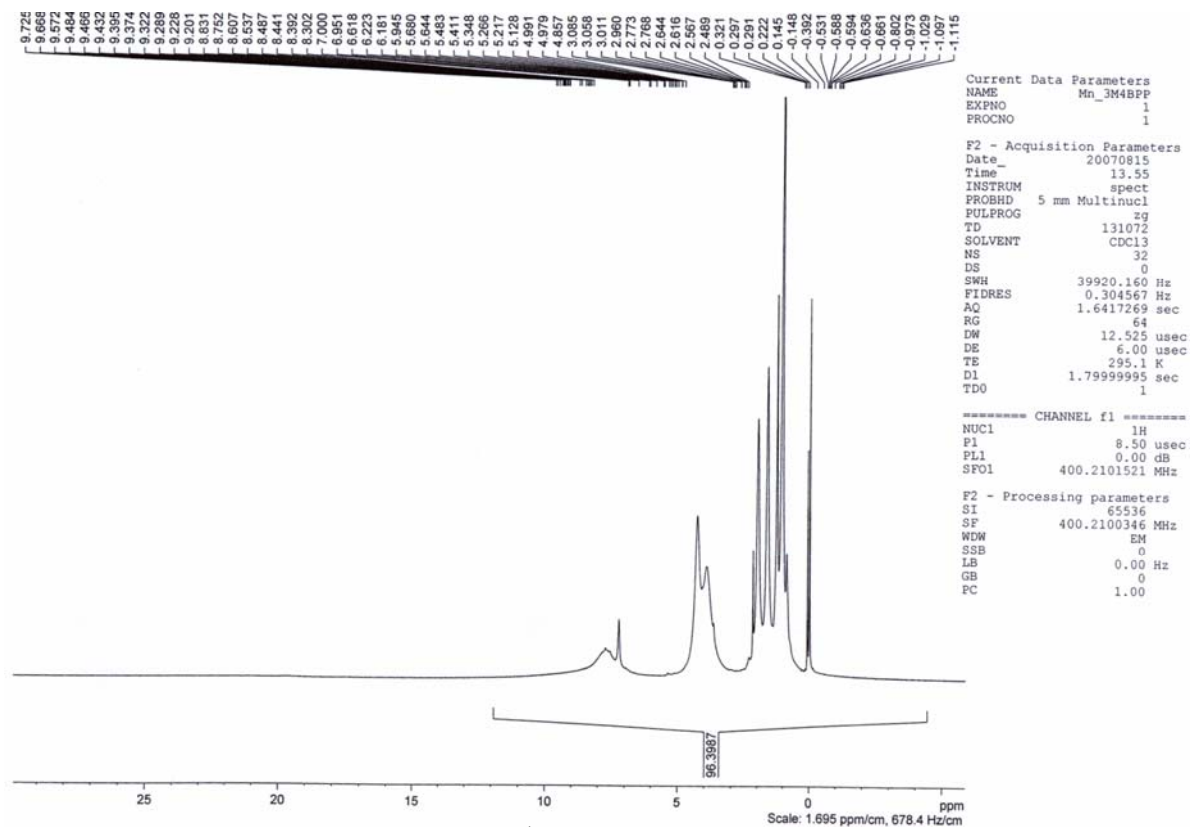
Espectro de RMN 1 H a 400 MHz de Mn(TBMP)
