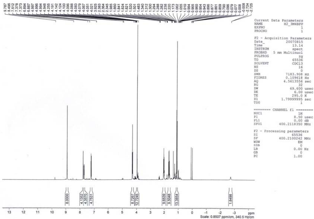
Espectro de RMN 1 H a 400 MHz de 27
