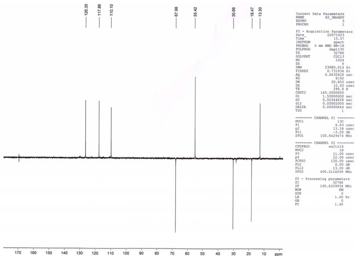
Espectro de PENDANT de 27
