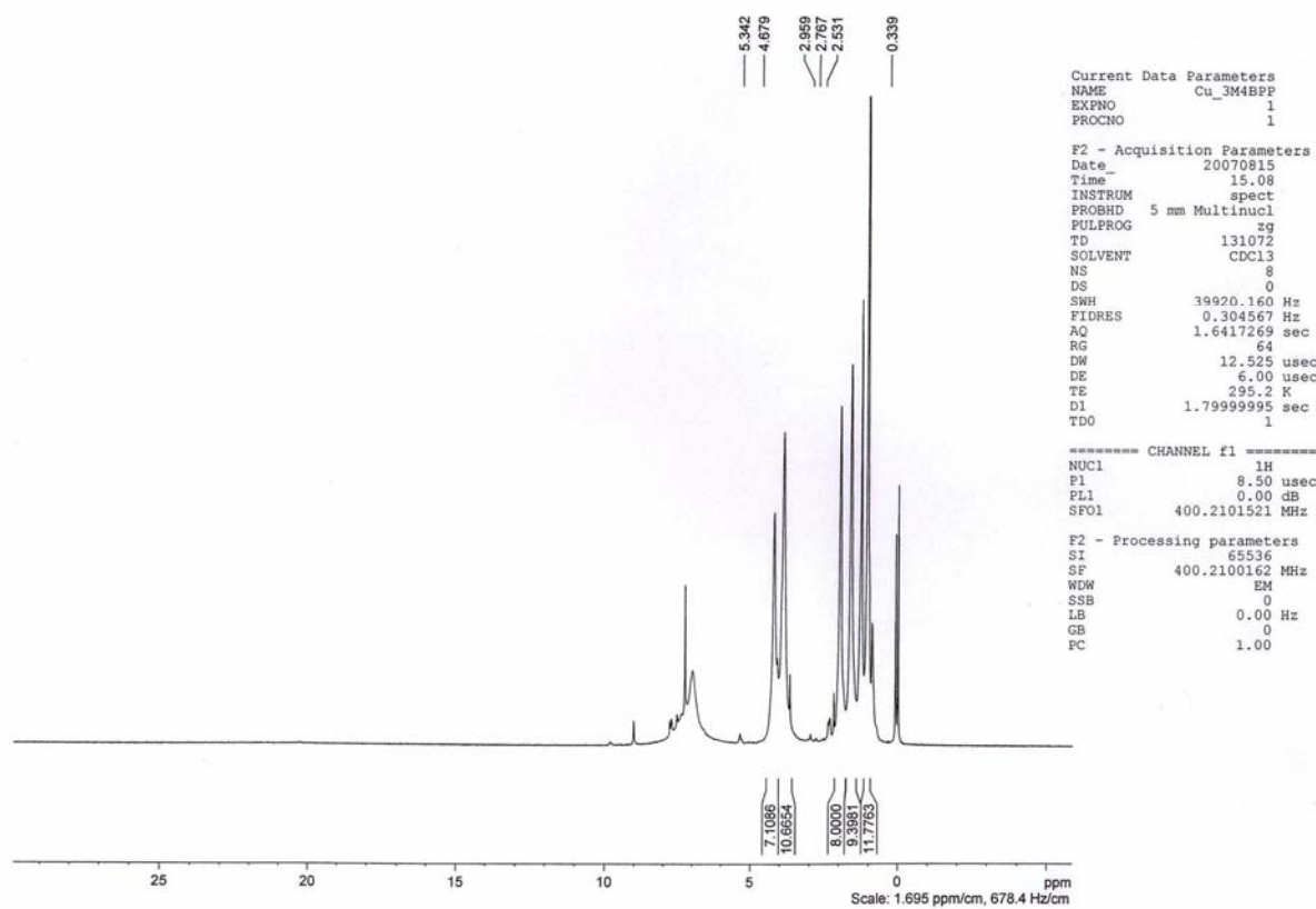
Espectro de RMN 1 H a 400 MHz de Cu(TBMPP)
