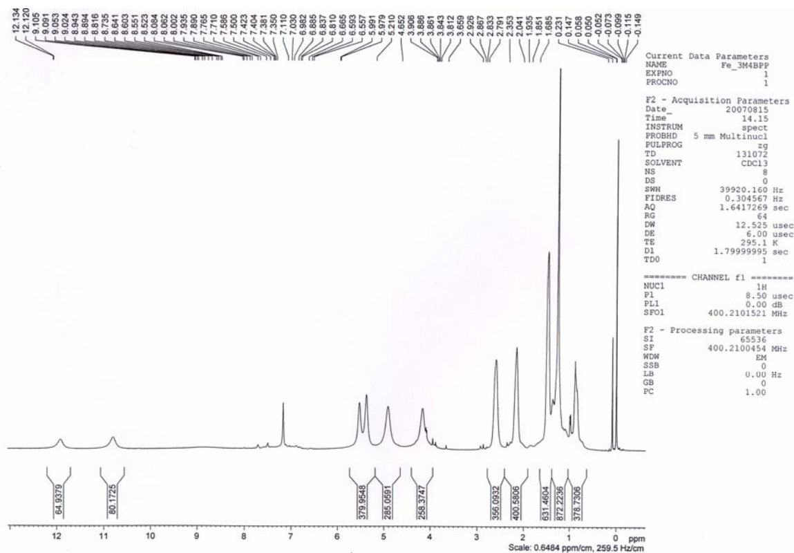
Espectro de RMN 1 H a 400 MHz de Fe(TBMPP)
