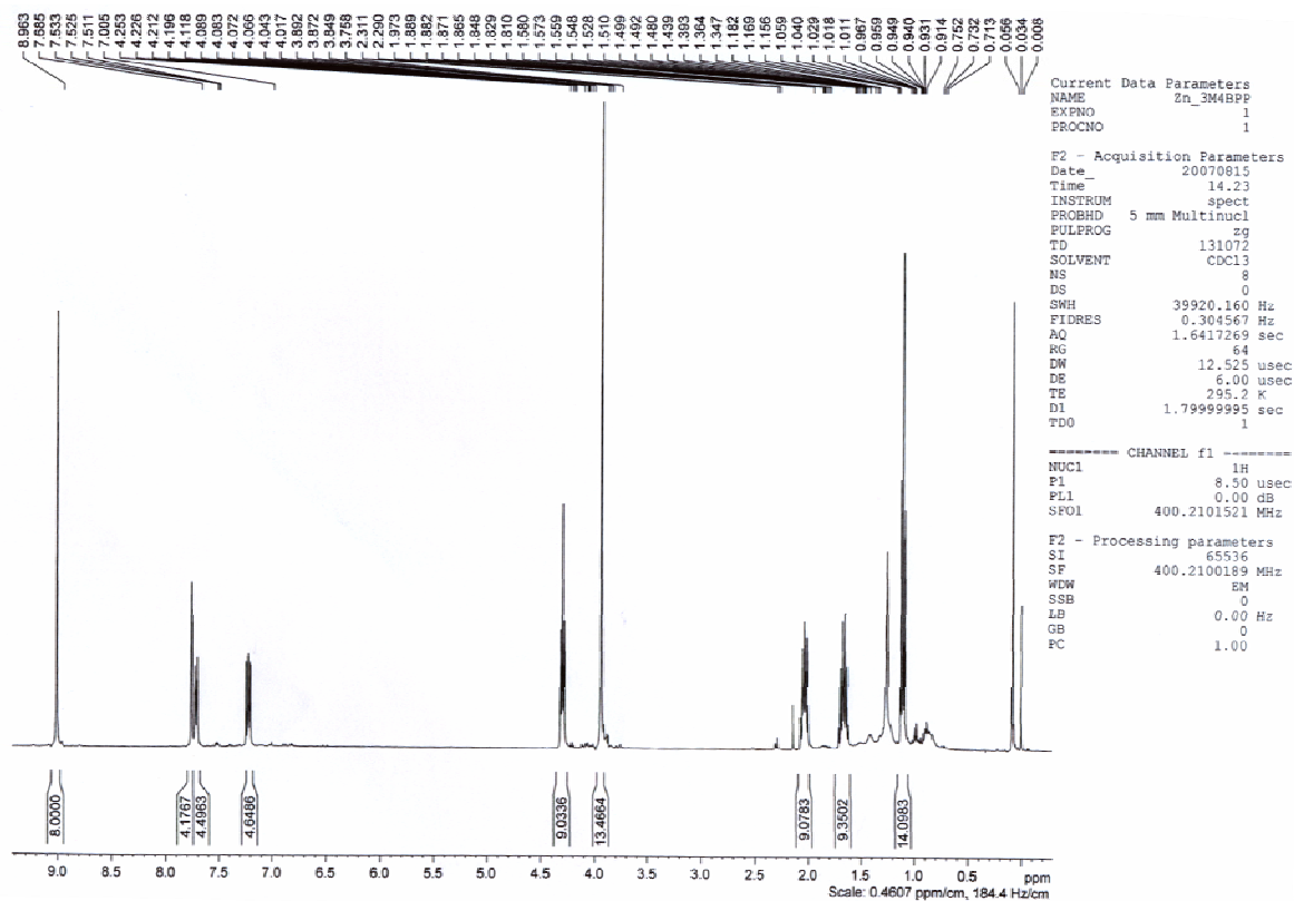
Espectro de RMN 1 H a 400 MHz de Zn(TBMP)
