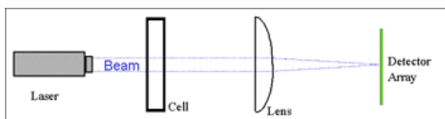
Figura 2 - Esquema da difração a laser no analisador de partículas
