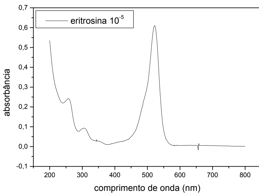
Figura 4 – Curva de absorção da eritrosina
