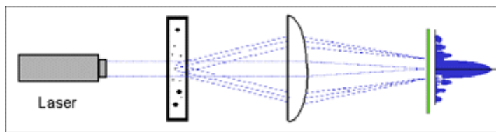
Figura 3 - Esquema da difração a laser no analisador de partículas
