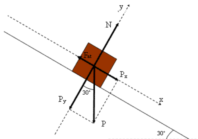
Figura 57 – Objeto em um plano inclinado
