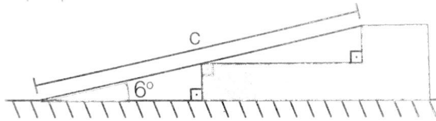
Figura 63 – Rampa seguindo a legislação
