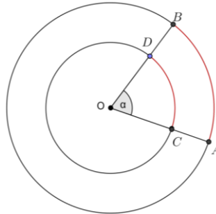
Figura 31 – Medida de um arco
