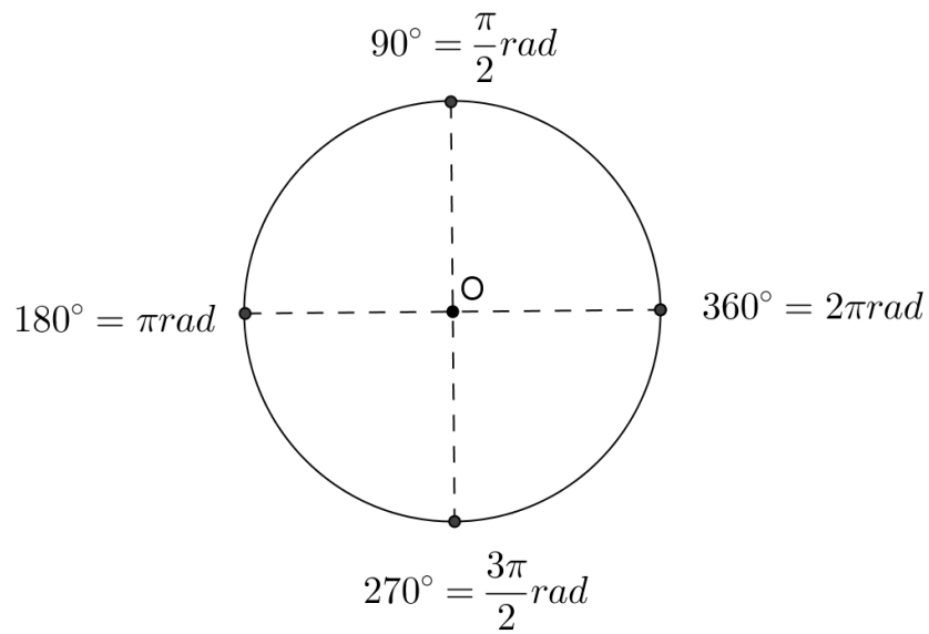
Figura 34 – Grau e radianos
