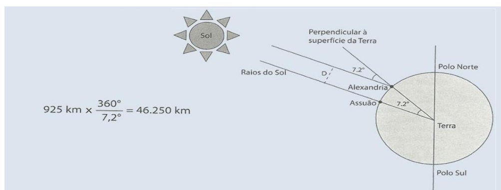
Figura 7 – Medida da Terra obtida por Erastótenes
