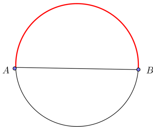
Figura 27 – Arcos com extremidades no diâmetro
