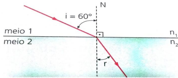
Figura 60 – Refração de um raio de luz
