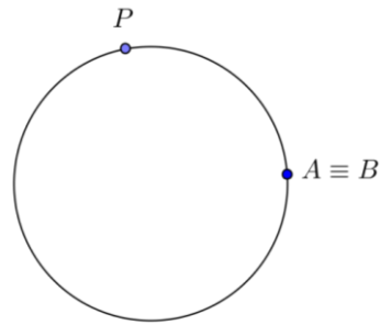
Figura 28 – Arco de uma volta
