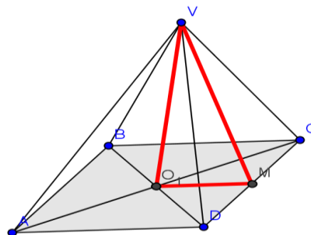
Figura 2 - Seqt egípcio
