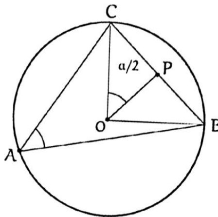
Figura 25 - Relação entre lado, seno do ângulo oposto e o raio da circunferência.
