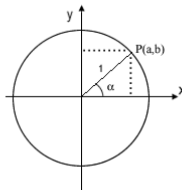
Figura 36 - Ciclo Trigonométrico
