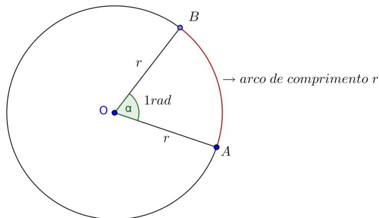
Figura 33 - Radianos
