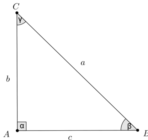
Figura 19 - Relação Fundamental
