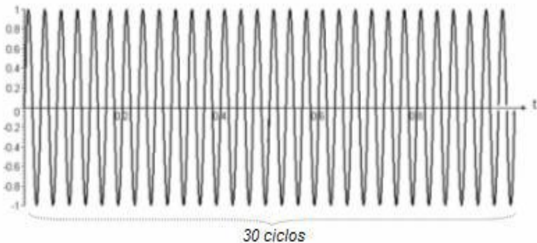
Figura 69 – Função y = \sin 60 \pi t
