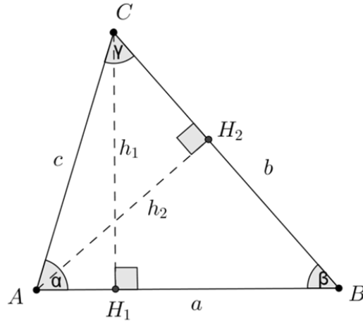
Figura 24 – Lei dos Senos
