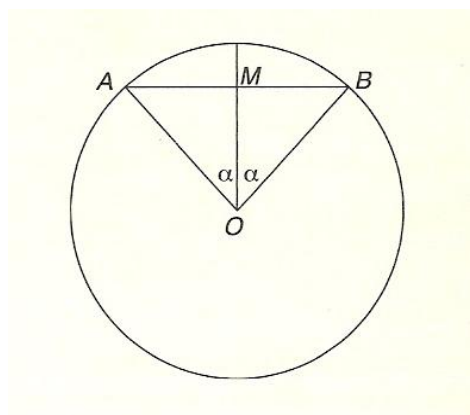
Figura 9 – Senos trigonométricos
