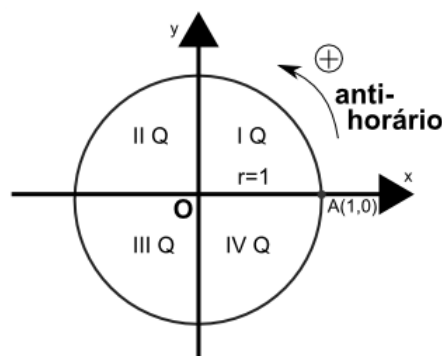
Figura 37 - Quadrantes
