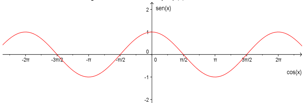
Figura 45 – Gráfico da função f(x) = \cos x .
