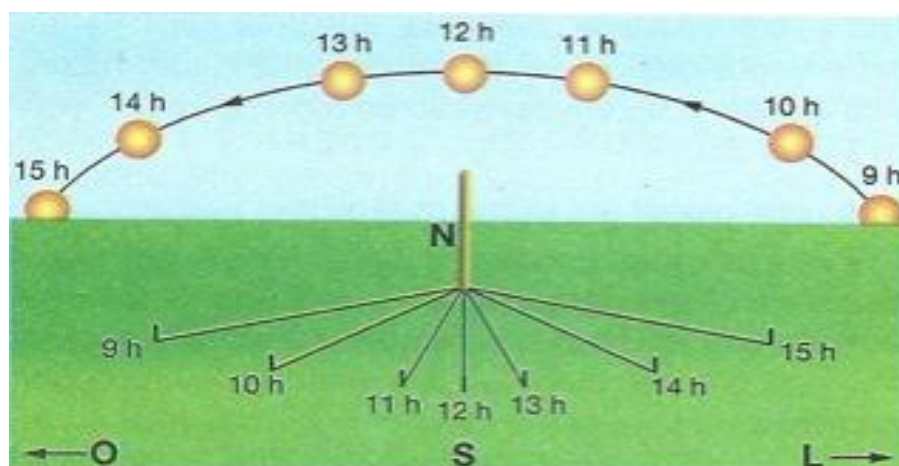
Figura 6 - Gnomon
