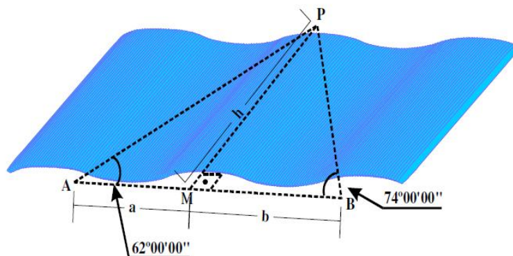
Figura 52: A Largura de um rio.
