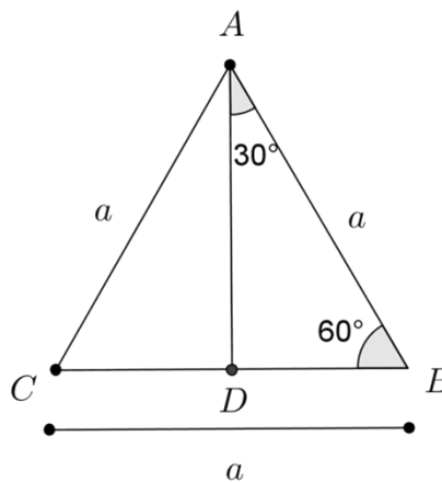
Figura 21 - Valores especiais para 30^\circ e 60^\circ
