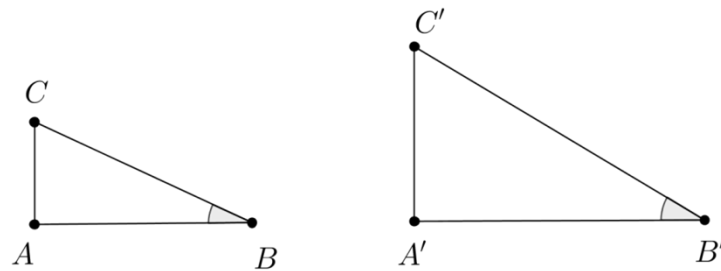
Figura 18 – Triângulos semelhantes
