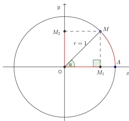
Figura 38 – Seno e cosseno de um arco
