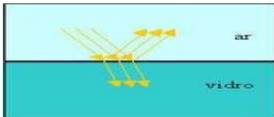
Figura 58 – Refração da luz
