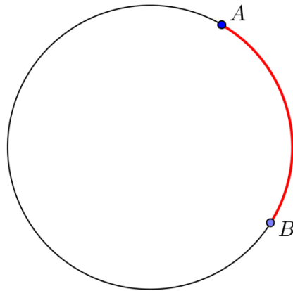
Figura 26 - Arco de circunferência
