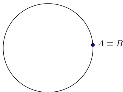
Figura 29 – Arco nulo
