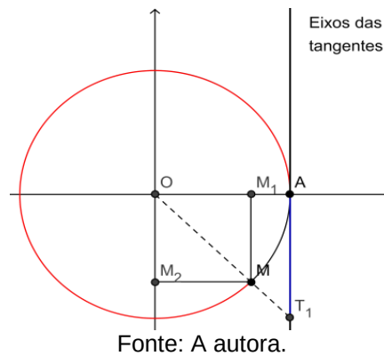
Figura 50 – Tangente no quarto quadrante
