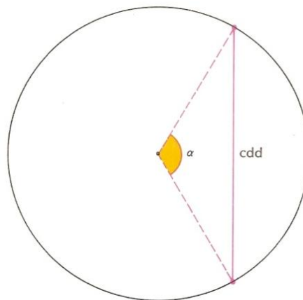
Figura 10 - Ângulo e corda segundo o Almajesto
