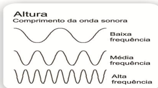
Figura 65 – Altura
