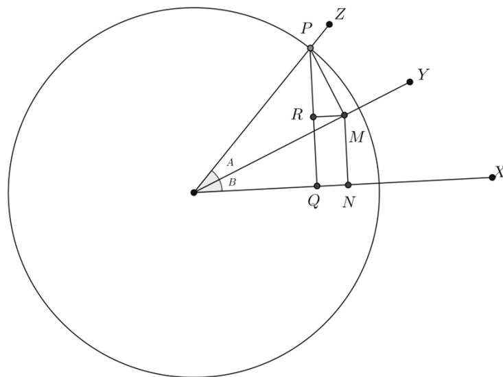
Figura 42 – Seno e cosseno da soma de ângulos
