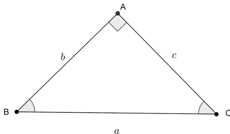
Figura 15 – Triângulo Retângulo
