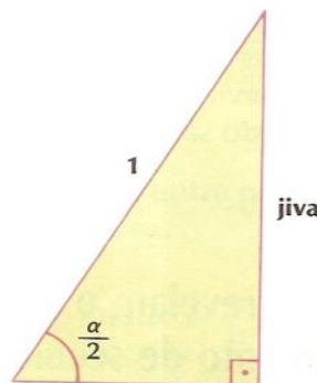
Figura 13 – Triângulo retângulo e a razão jiva
