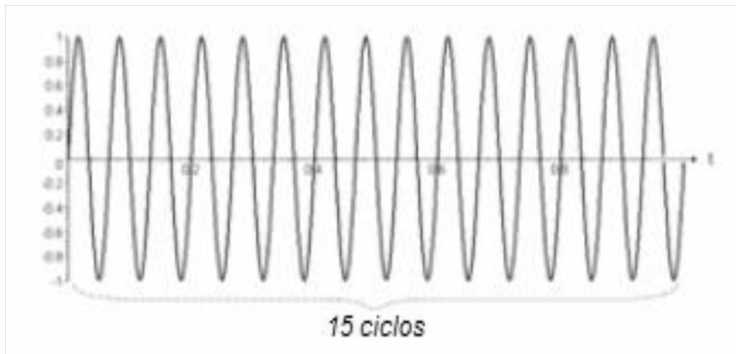
Figura 68 – Função y = \sin 30 \pi t
