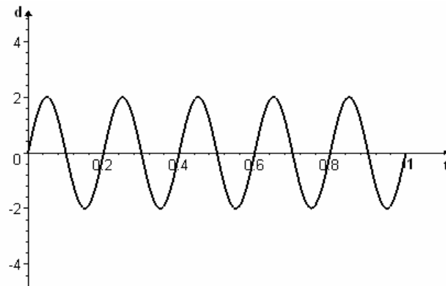
Figura 71 – Amplitude de y = 2 \cdot \text{sen } 10\pi t
