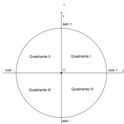
Figura 39 – Sinais nos quadrantes
