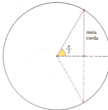
Figura 11 – Ângulo e corda segundo Siddhanta
