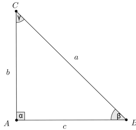
Figura 20 – Relações trigonométricas
