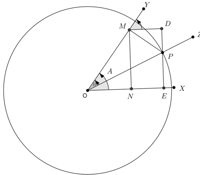
Figura 43 – Seno e cosseno da diferença de ângulos
