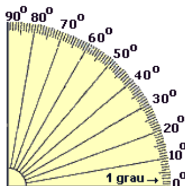
Figura 32 – Grau
