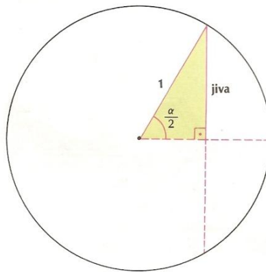
Figura 12 – Jiva e o círculo de raio unitário
