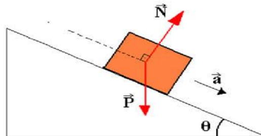
Figura 55 – Plano Inclinado
