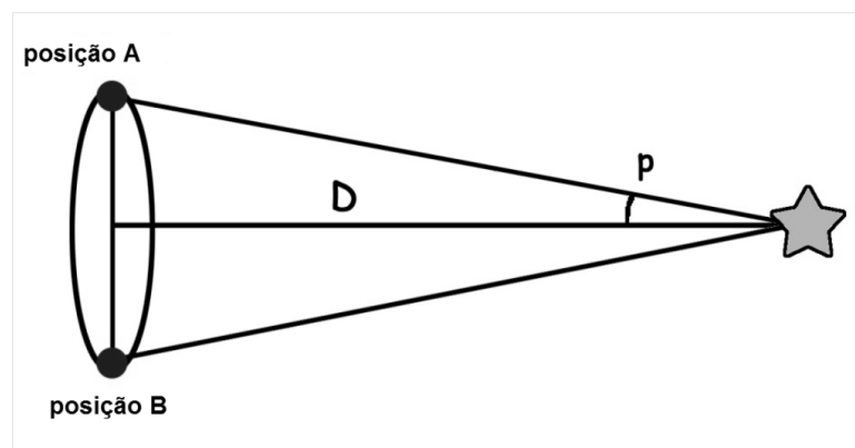
Figura 53 - Distância da estrela
