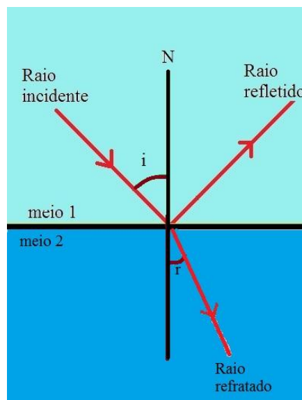
Figura 59 - Refração da Luz
