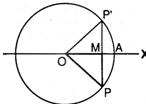
Figura 41 – Ângulos negativos.
