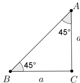
Figura 22 – Valores especiais para 45^\circ
