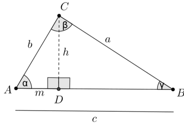
Figura 23 – Lei dos Cossenos
