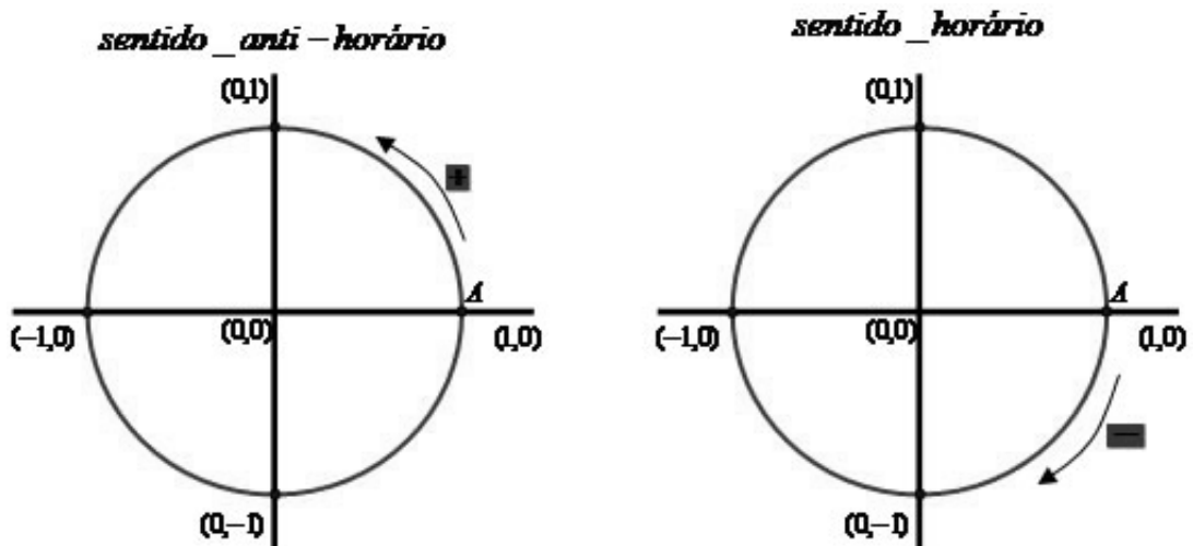
Figura 35 - Sentido do arco
