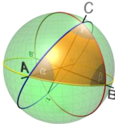
Figura 8 – Trigonometria esférica
