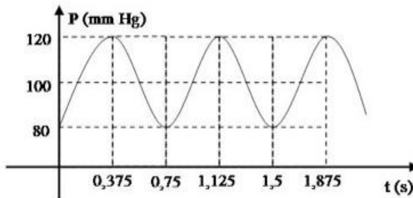
Figura 72 - Representação dos batimentos cardíacos de uma pessoa
