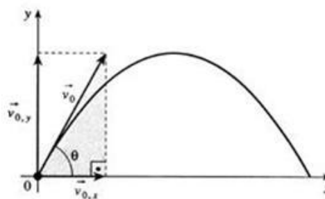
Figura 54 – Lançamento oblíquo
