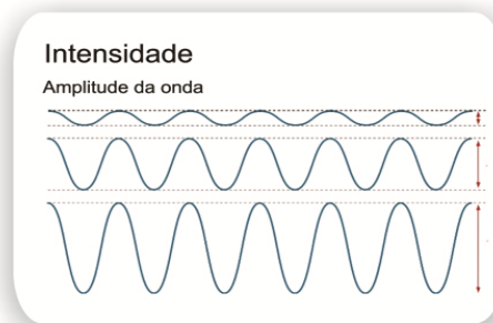
Figura 64 – Intensidade
