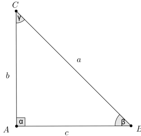
Figura 17 – Razões trigonométricas
