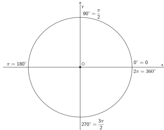
Figura 40 – Valores comuns
