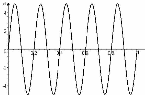
Figura 70 – Amplitude de y = 5 \cdot \text{sen } 10\pi t
