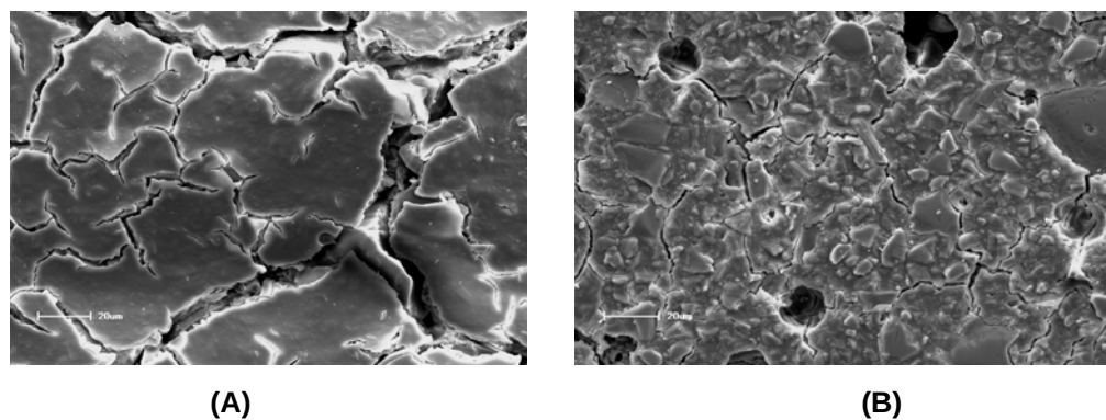
Figura 21 – Fotomicrografia do cimento de ionômero de vidro convencional Maxxion R, antes (A) (Ra 1,18 \mu\text{m} ) e após (B) (Ra 4,03 \mu\text{m} ) escovação simulada
