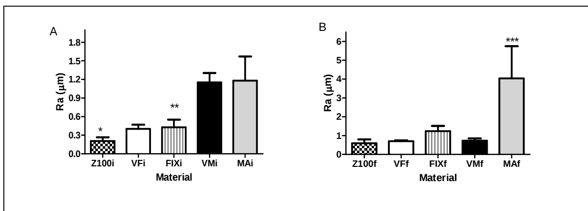
Figura 14- Média e erro padrão da rugosidade dos diferentes materiais (Z100- Resina Z100; VF- Vitrofil; FIX- Fuji IX; VM- Vitro Molar; MA- Maxxion). (A) Rugosidade inicial, diferenças significativas entre os grupos ( p < 0,0001 ). * p < 0,001 com VM e MA; ** p < 0,05 com VM e MA. (B) Rugosidade final, diferenças significativas entre os grupos ( p < 0,05 – ANOVA); *** p < 0,05 com VF, VM e Z100. ANOVA 1 critério com pós teste de Tukey.
