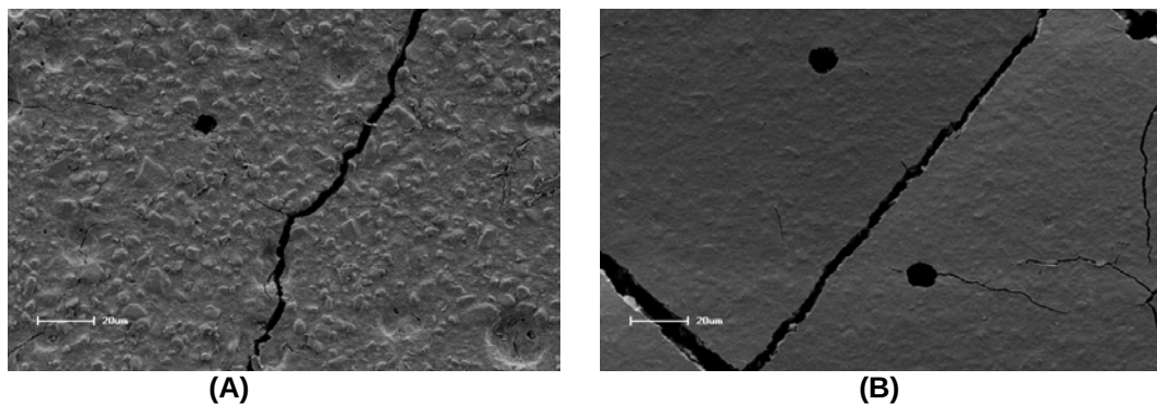
Figura 20 – Fotomicrografia do cimento de ionômero de vidro de alta viscosidade Vitro Molar, antes (A) (1,15 \mu\text{m} ) e após (B) (Ra 0,73 \mu\text{m} ) escovação simulada
