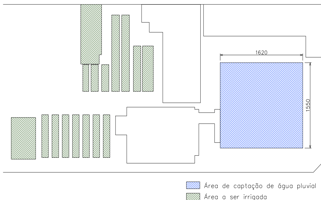
Figura 1 – Representação das edificações com 715,39m 2 de área construída e o arranjo dos canteiros existentes. (Fonte: Autores)
