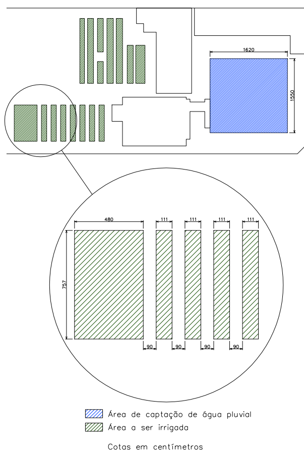
Figura 4 – Representação da nova disposição sugerida dos canteiros. (Fonte: Autores)
