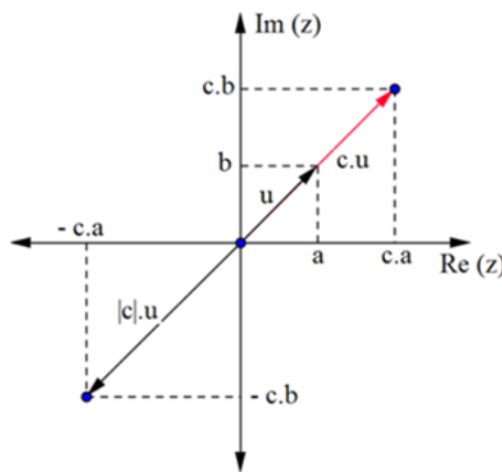
Figura 6: produto do complexo u pelo número real c Fonte: a autora
