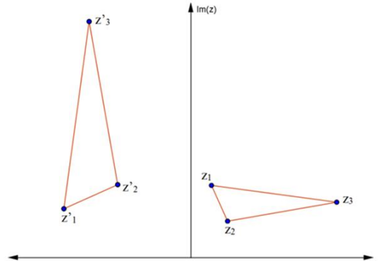
Figura 36: triângulos semelhantes de mesma orientação Fonte: a autora
