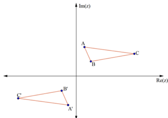
Figura 25: rotação de ABC 180^\circ em torno da origem
