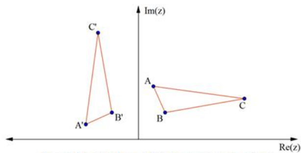
Figura 24: rotação de ABC 90^\circ em torno da origem
