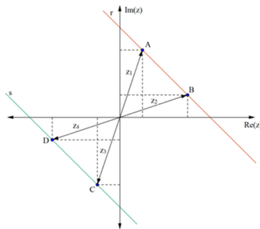
Figura 33: retas paralelas no plano complexo Fonte: a autora
