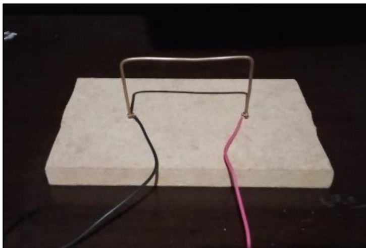
Figura 28 - Aparato Experimento de Oersted.
