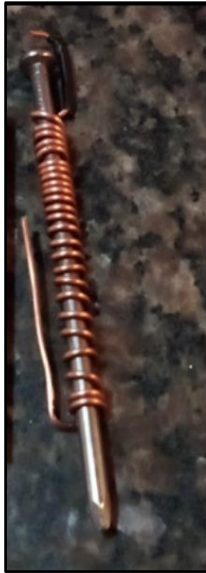
Figura 11 – Eletroímã.
