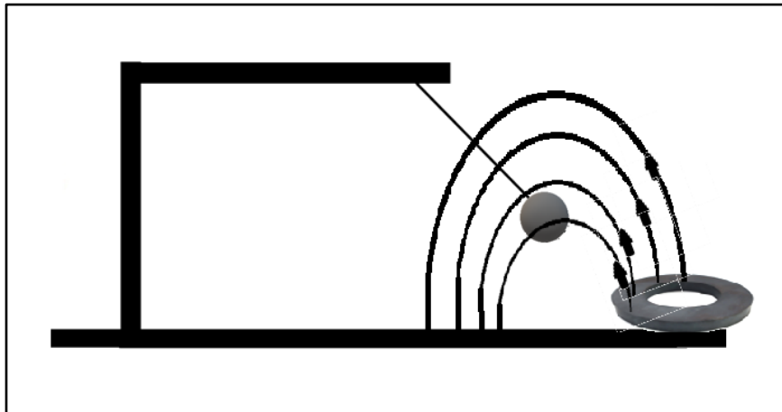
Figura 2 – Esquema da montagem do aparato da Tesoura de Gauss representando algumas linhas de campo, geradas pelo ímã de anel (apenas parte das linhas de campo foram representadas na figura).
