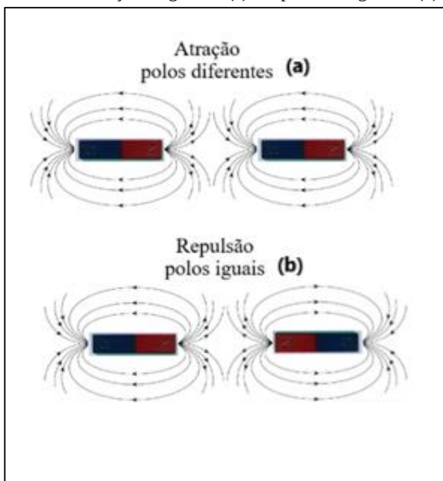
Figura 5 - Representação das linhas de campo magnético entre dois ímãs de barra em duas situações: atração magnética (a) e repulsão magnética (b).
