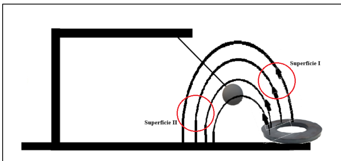
Figura 16 - Esquema da montagem representando algumas linhas de campo, geradas pelo ímã de anel (apenas parte das linhas de campo foram representadas na figura) representando as Superfícies Gaussianas I e II.
