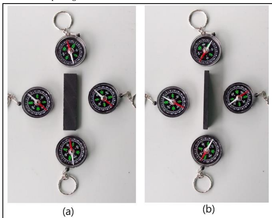
Figura 7 – Orientação do campo magnético de um ímã em barra, usando bússolas. Aqui foi considerado apenas o campo magnético ao redor do ímã.
