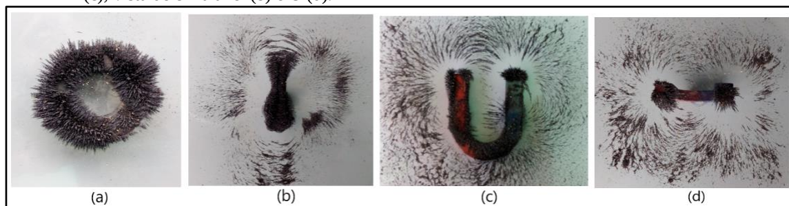
Figura 11 - Representação das linhas de campo com o uso da limalha de ferro: vista lateral – anel (a) e U (c), vista de cima anel (b) e U (d).
