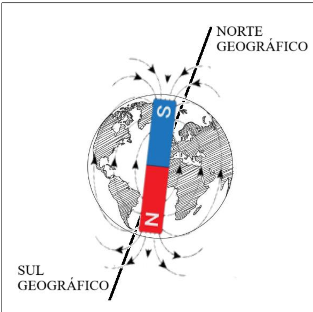
Figura 8 - Representação do campo magnético terrestre, polos magnéticos e polos geográficos da Terra.
