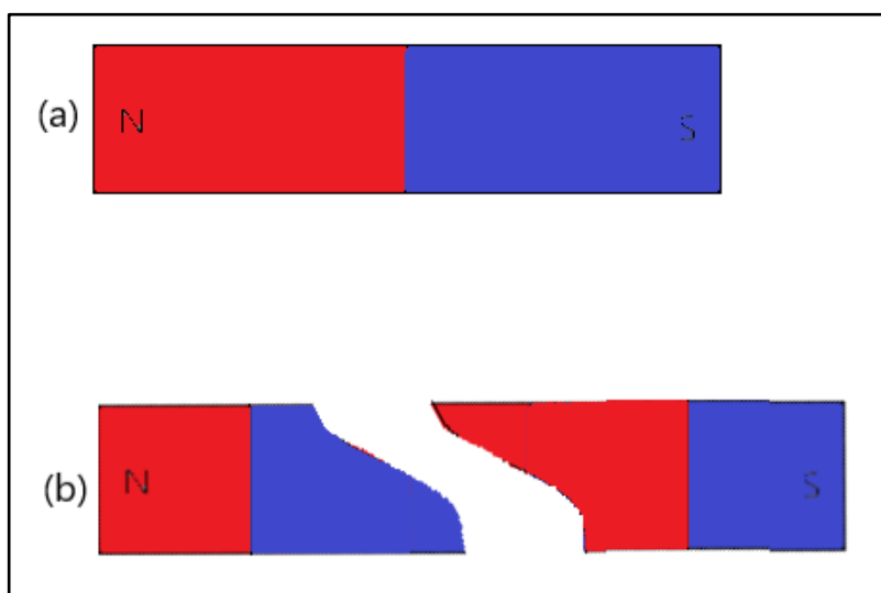
Figura 12 - Representação dos polos magnéticos de um ímã de barra: antes de ser partido(a), após ser partido e sem levar em consideração a interação magnética entre os pedaços do ímã (b).
