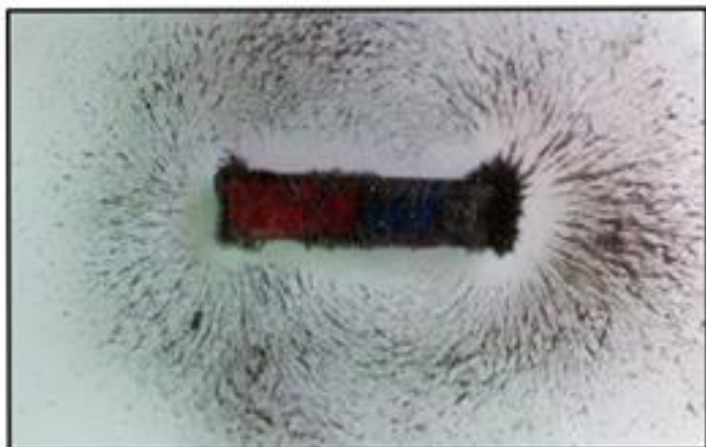
Figura 17 - Representação das linhas de campo magnético do ímã de barra com o uso da limalha de ferro.
