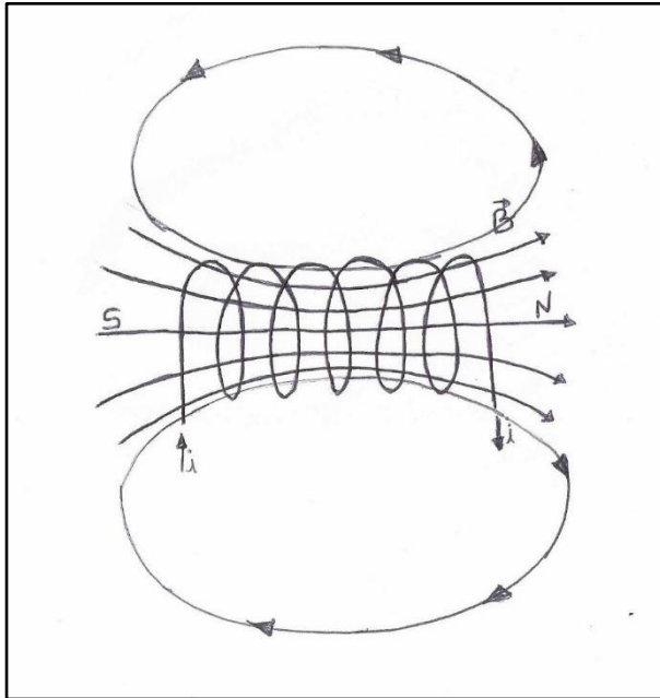
Figura 12 - Representação esquemática de um solenoide e as linhas de campo no interior do mesmo.
