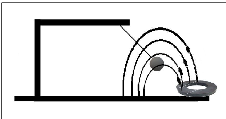
Figura 4 – Aparato da Base da Tesoura de Gauss representando algumas linhas de campo, geradas pelo ímã de anel (apenas parte das linhas de campo foram representadas na figura).
