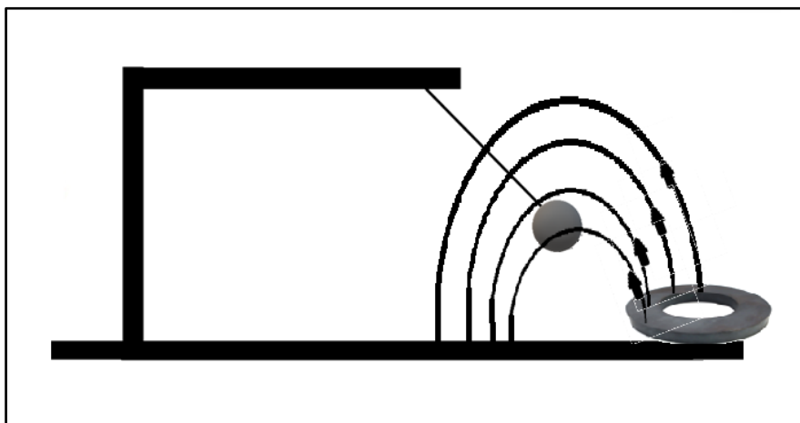
Figura 3 – Aparato da Base da Tesoura de Gauss representando algumas linhas de campo, geradas pelo ímã de anel (apenas parte das linhas de campo foram representadas na figura).
