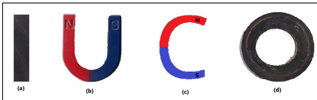
Figura 6 - Representação dos ímãs em formato de: barra (a), u (b), c (c) e anel (d).
