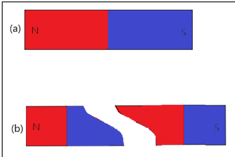
Figura 10 – Representação dos polos magnéticos de um ímã de barra: antes de ser partido(a), após ser partido e sem levar em consideração a interação magnética entre os pedaços do ímã (b).
