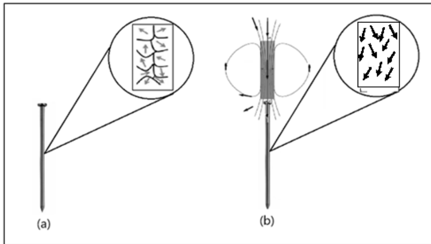
Figura 19 – Representação do processo de magnetização de um prego, material ferromagnético, com o uso de um ímã de barra, campo magnético externo, e na ampliação representação microscópica dos domínios magnéticos: antes do processo (a) e depois do processo (b).
