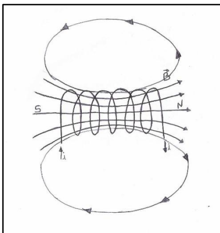
Figura 14 - Representação esquemática de um solenoide e as linhas de campo no interior do mesmo.
