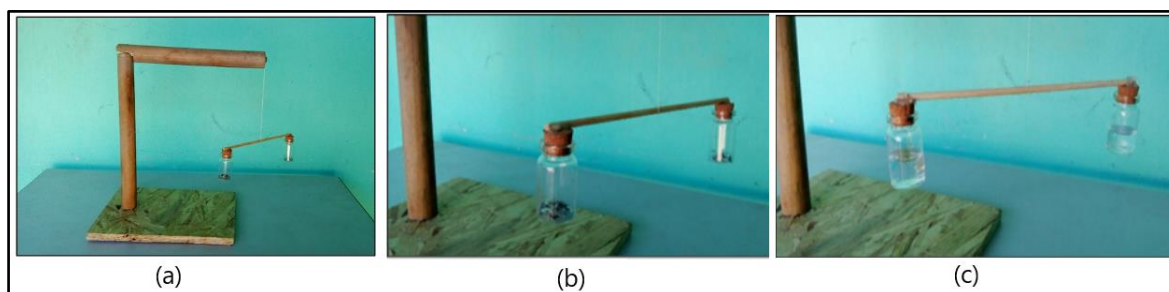
Figura 27 - Aparato para materiais paramagnéticos e diamagnéticos.
