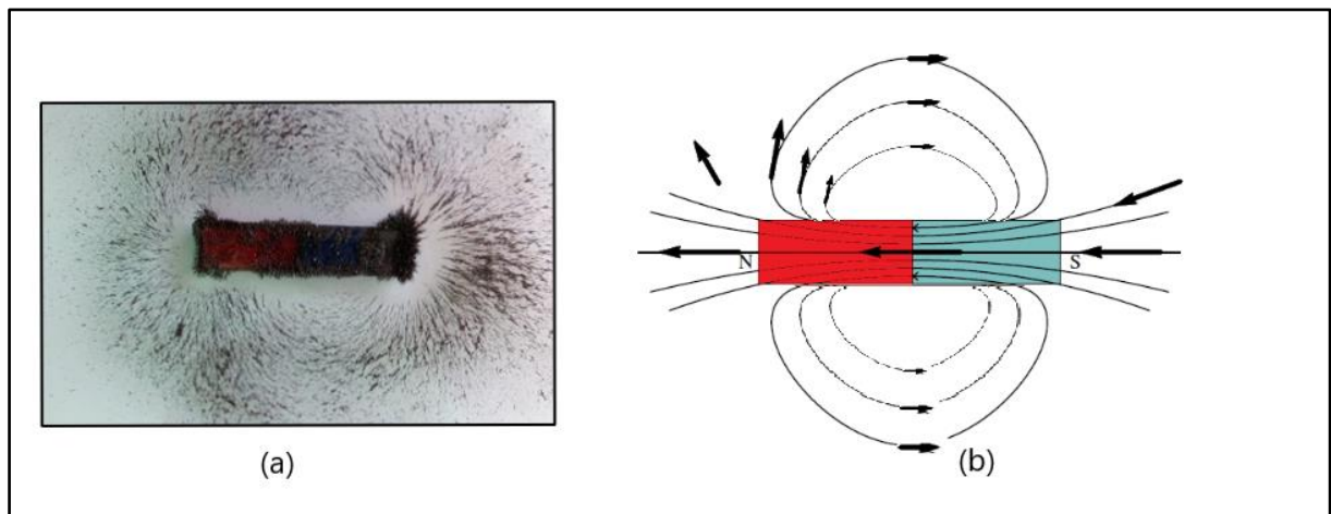
Figura 8 – Representação das linhas de campo magnético em um ímã de barra com o uso de limalha de ferro (a) e vetorial por meio das linhas de campo e campo magnético (b).
