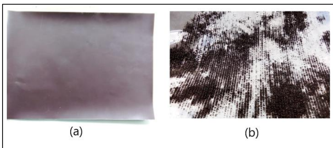
Figura 7 - Ímã em formato de folha (a), ímã de folha com limalha (b).
