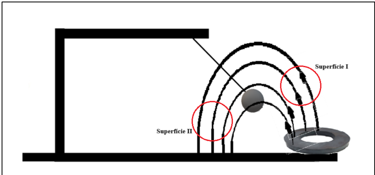
Figura 14 – Esquema da montagem representando algumas linhas de campo, geradas pelo ímã de anel (apenas parte das linhas de campo foram representadas na figura) representando as Superfícies Gaussianas I e II.
