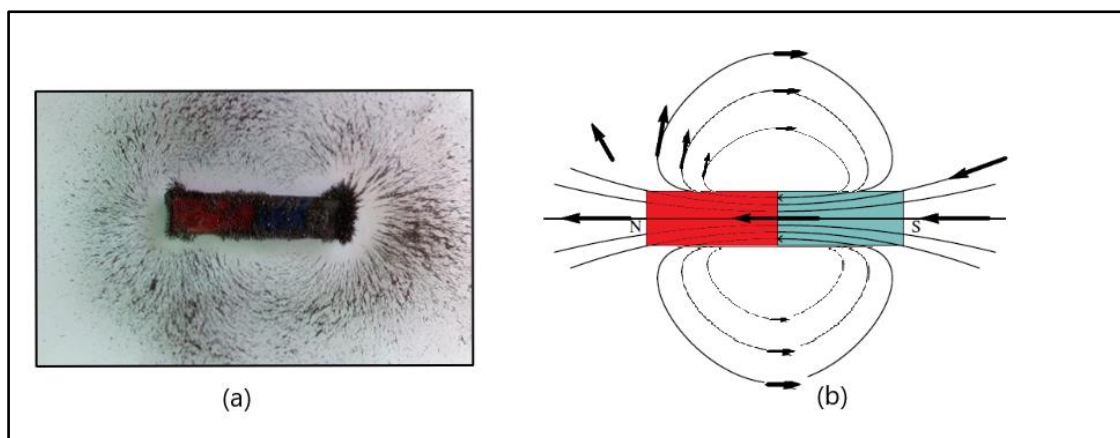
Figura 10 - Representação das linhas de campo magnético em um ímã de barra com o uso de limalha de ferro (a) e vetorial por meio das linhas de campo e campo magnético (b).
