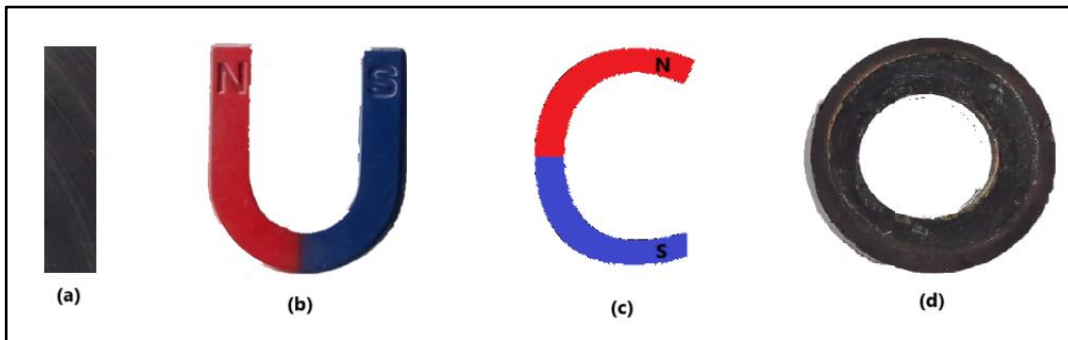
Figura 4 – Representação dos ímãs em formato de: barra (a), u (b), c (c) e anel (d).
