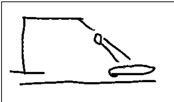
Figura 2 - Representação das linhas de campo
