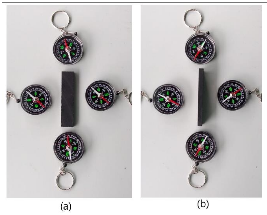
Figura 9 - Orientação do campo magnético de um ímã em barra, usando bússolas. Aqui foi considerado apenas o campo magnético ao redor do ímã.
