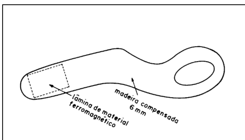
Figura 23 - Molde para a Tesoura de Gauss.
