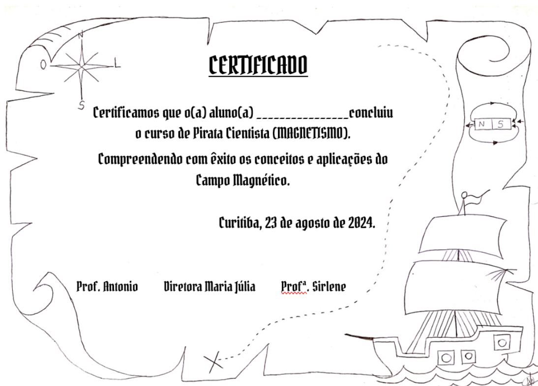
Figura 41 - Certificado Pirata Cientista.
