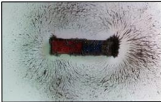
Figura 15 – Representação das linhas de campo magnético do ímã de barra com o uso da limalha de ferro.
