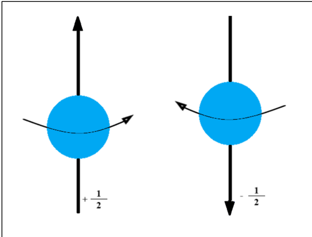
Figura 16 – Representação do spin do elétron em dois estados possíveis.
