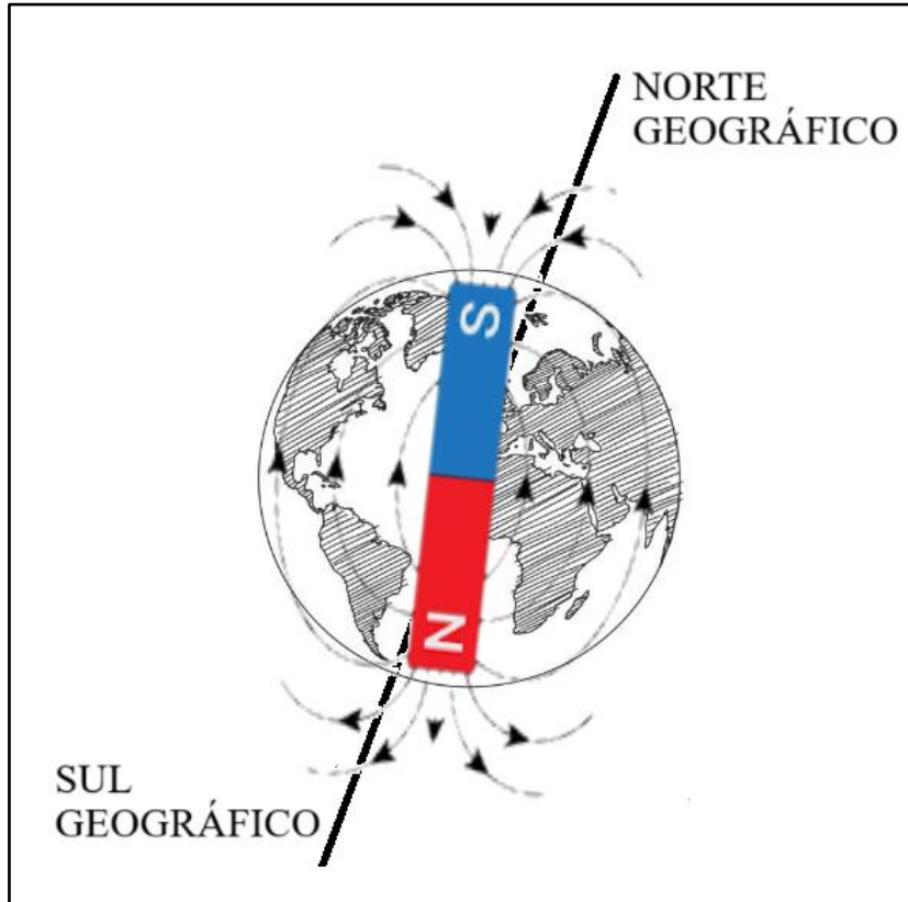
Figura 6 – Representação do campo magnético terrestre, polos magnéticos e polos geográficos da Terra.
