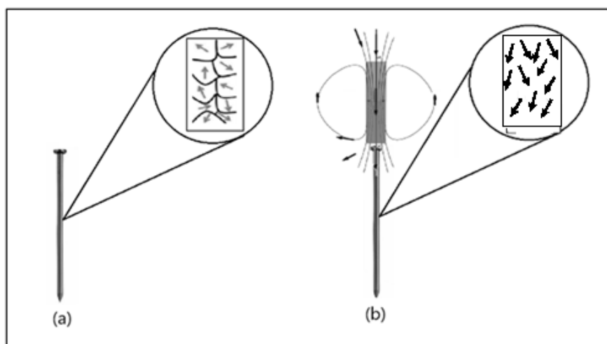
Figura 21 - Representação do processo de magnetização de um prego, material ferromagnético, com o uso de um ímã de barra, campo magnético externo, e na ampliação representação microscópica dos domínios magnéticos: antes do processo (a) e depois do processo (b).
