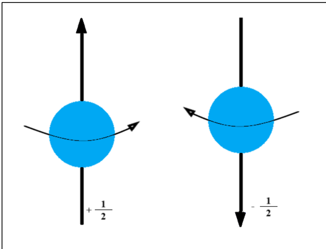
Figura 18 - Representação do spin do elétron em dois estados possíveis.
