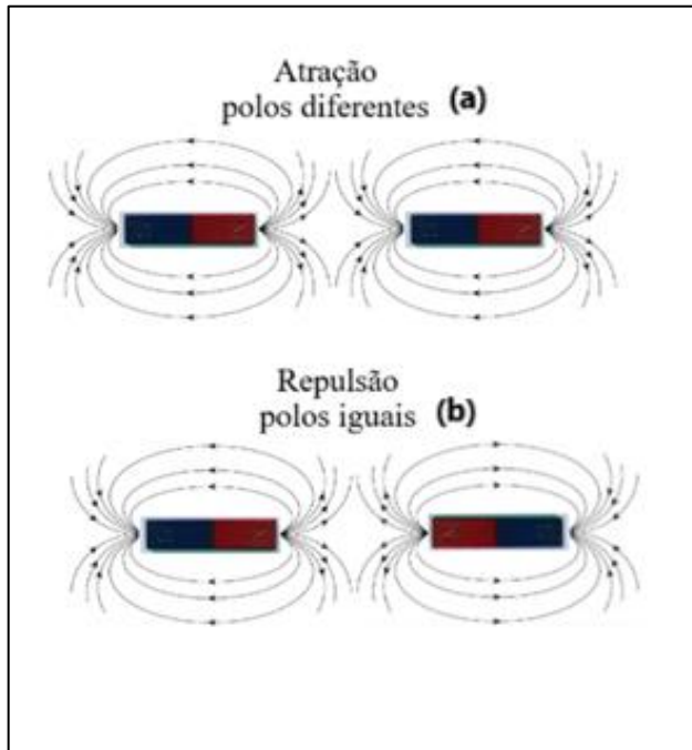
Figura 3 - Representação das linhas de campo magnético entre dois ímãs de barra em duas situações: atração magnética (a) e repulsão magnética (b).
